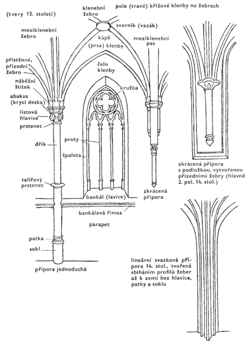
Články gotického klenutého interiéru
